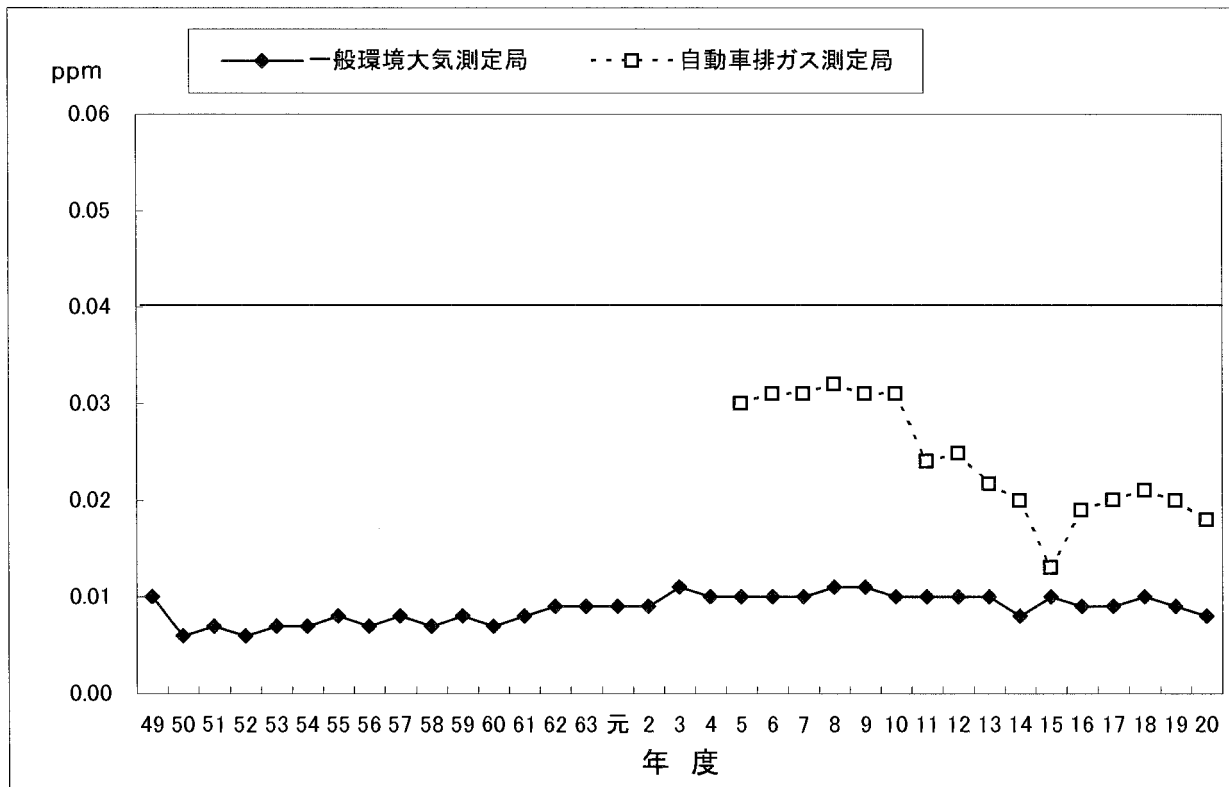
二酸化窒素年平均値の経年変化 (一般局：有効測定局数平均、自排局1局)
