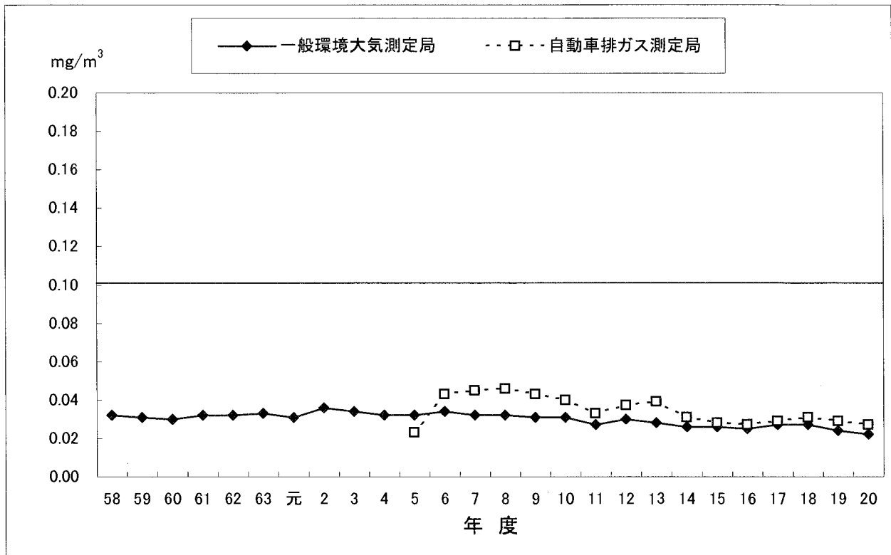
浮遊粒子状物質年平均値の経年変化 (一般局：有効測定局数平均、自排局1局)
