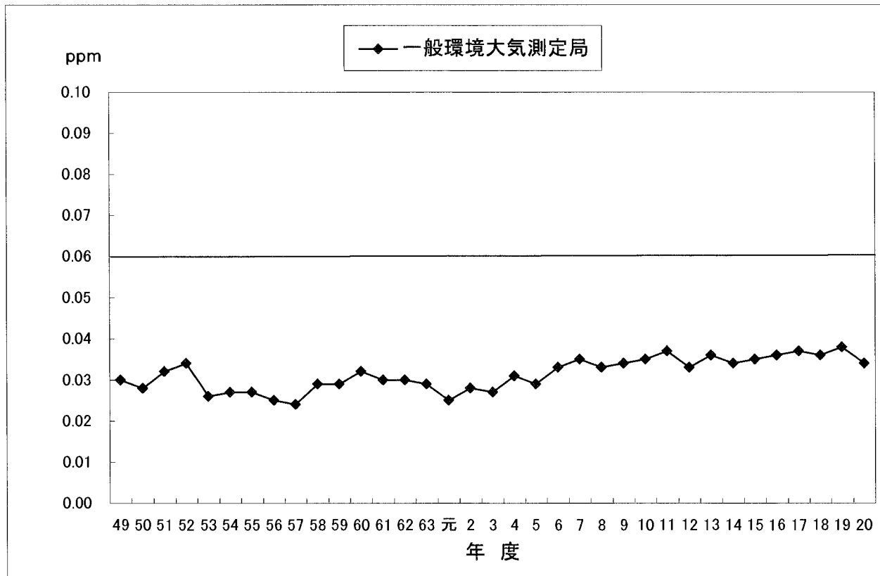
光化学オキシダント昼間の1時間値の年平均 (有効測定局数平均)
