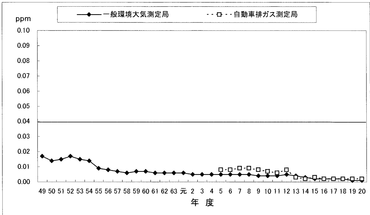
二酸化いおう年平均値の経年変化 (一般局：有効測定局数平均、自排局1局)
